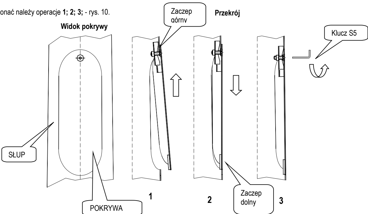
Rys. 10 Montaż pokrywy wnętrza kablowej.
