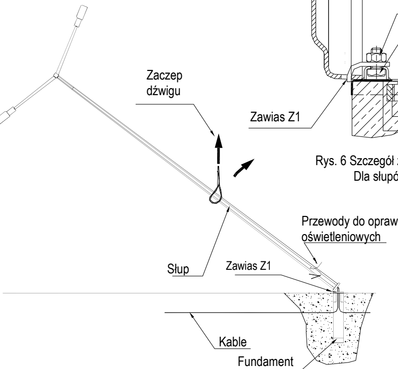
Rys. 7 Ustawianie słupa na zawiasie
